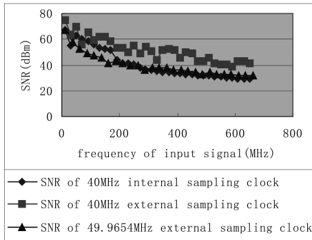
图2 不同采样时钟的SNR
