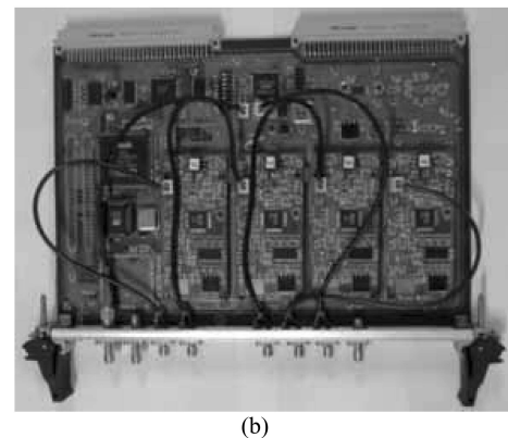
图 1 (a) 系统框图; (b) 数据采集板卡实物图
