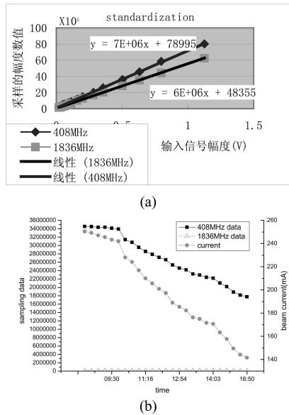
图 5 (a) 系统两路标定; (b) 测试数据、流强随时间的变化关系
