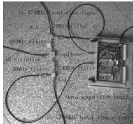
图4 束长测量设备图
