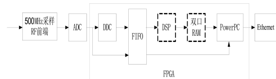
图 6 改进系统框图
